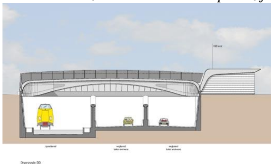
Doorsnede van de tunnel
